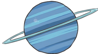
Uranus
